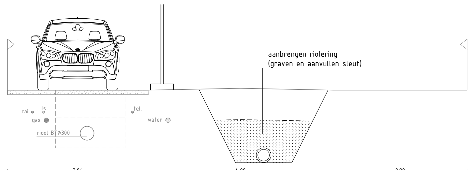
fase 3, aanleg riolering schaal 1:50
