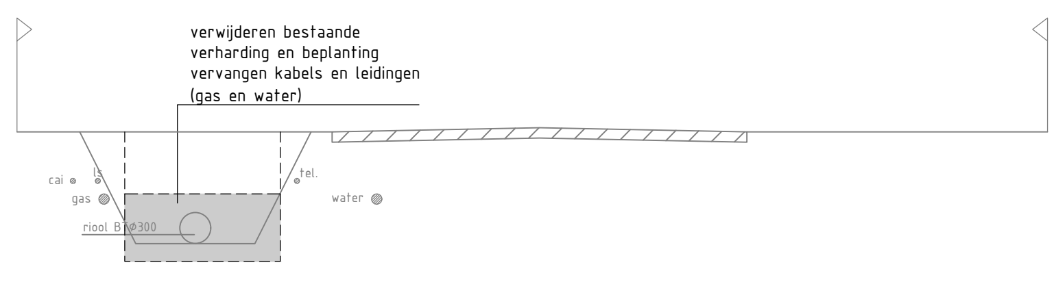
fase 1, vervangen kabels en leidingen schaal 1:50
