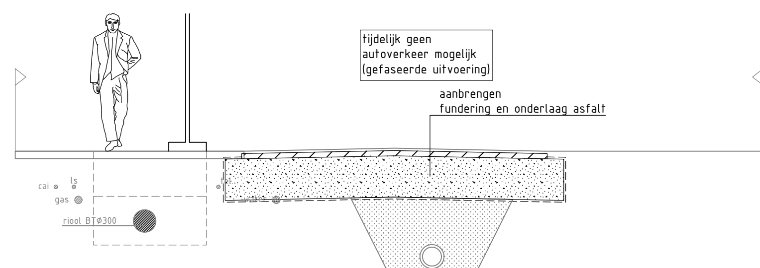
fase 4, aanleg fundering en onderlaag asfalt schaal 1:50
