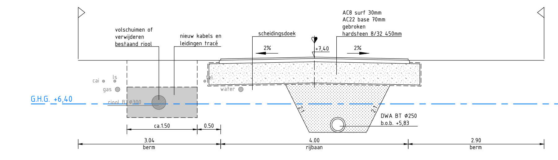
dwarsprofiel A-A schaal 1:50
