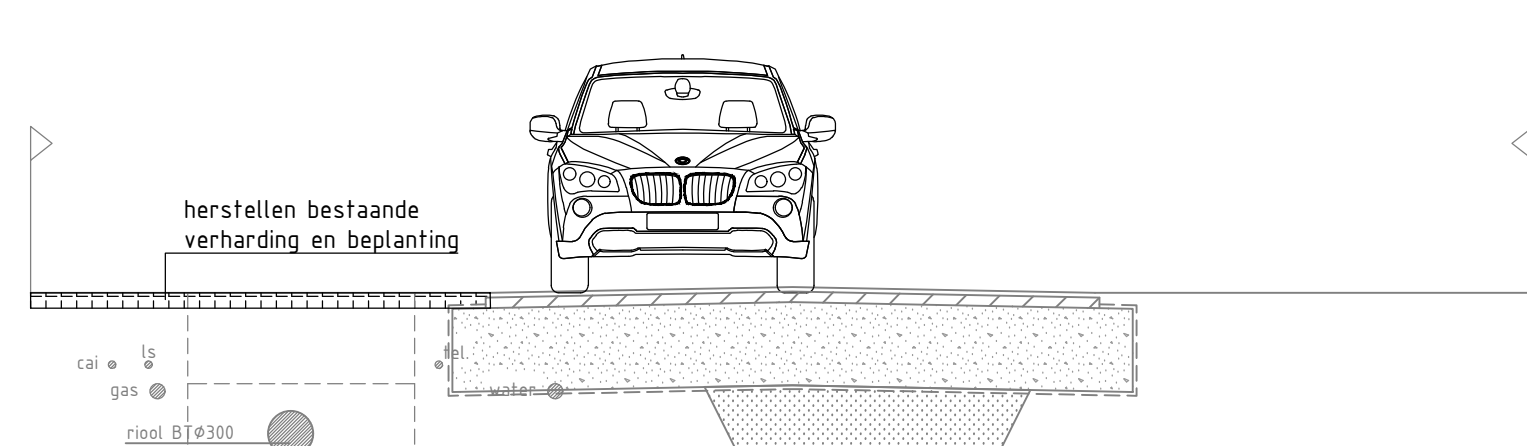
fase 4, aanleg fundering en onderlaag asfalt schaal 1:50
