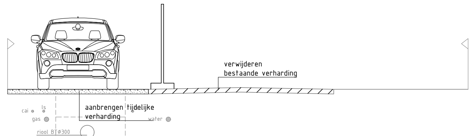
fase 1, vervangen kabels en leidingen schaal 1:50
