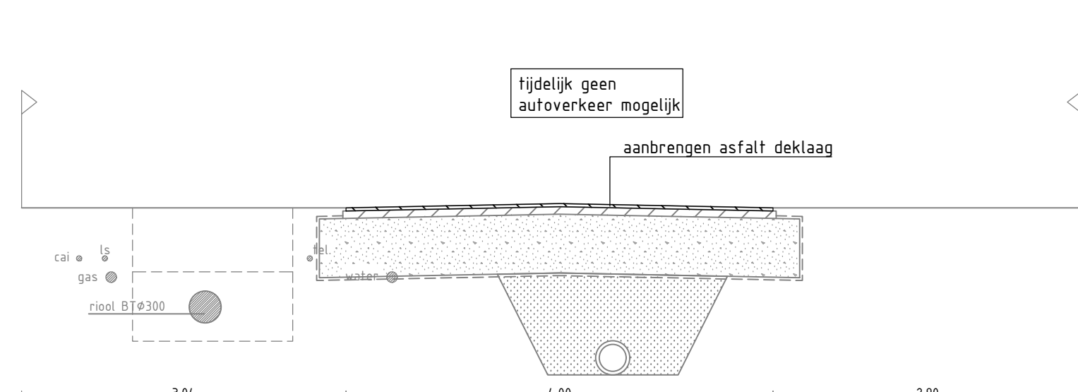
fase 6, aanleg deklaag asfalt schaal 1:50
